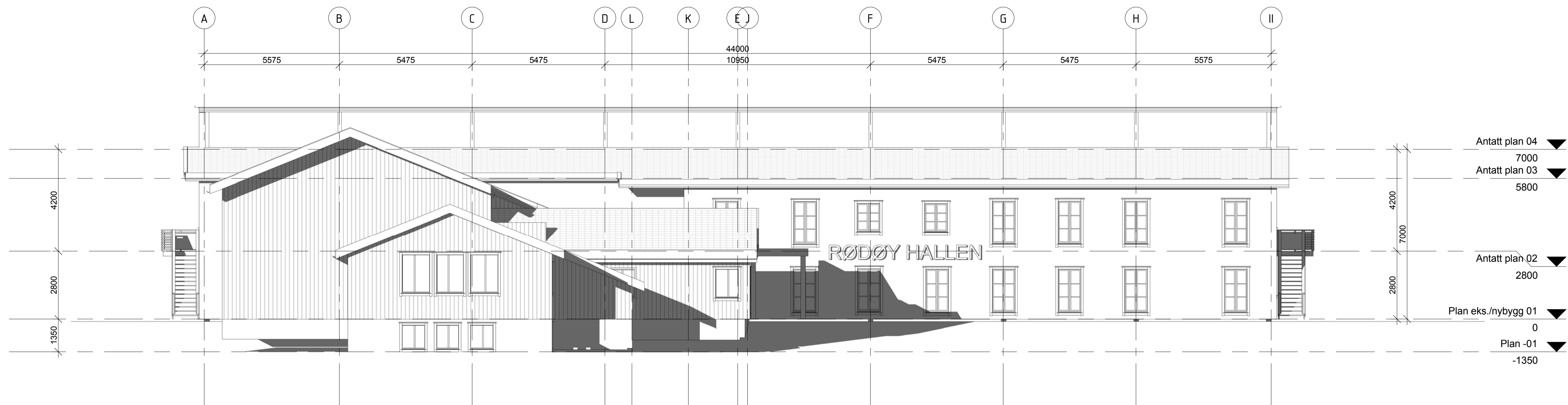
Fasade Sør 1 : 100
