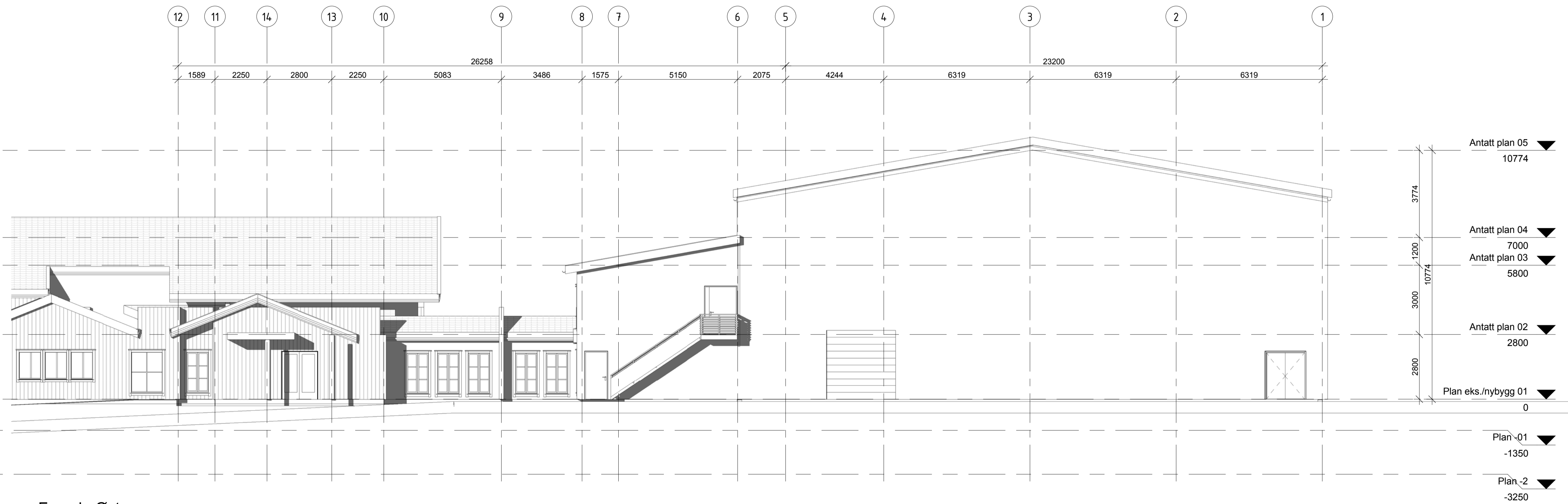
Fasade Øst 1 : 100
