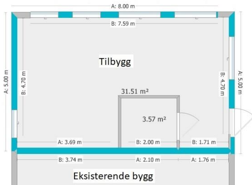
Figur 3 - Planskisse
