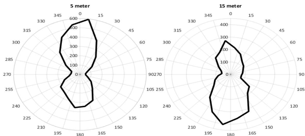
Figur 3: Vanntransport ( \text{m}^3/\text{m}^2/\text{dag} ) for hver 15^\circ sektor på hhv. 5 og 15 meters dyp ved Prestvika i perioden 04.04.2023–10.05.2023 (Nergaard, 2023).
