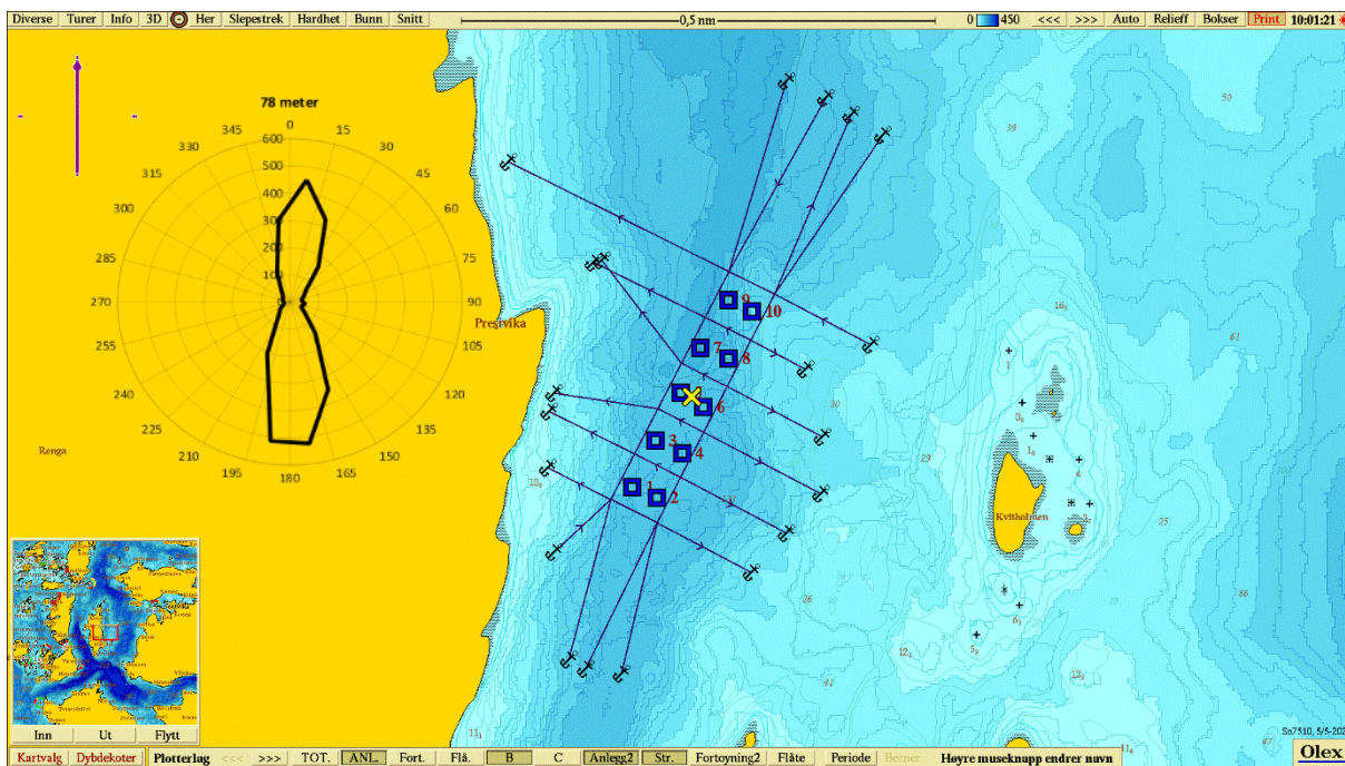
Figur 3: Kartet viser anleggsplassering sammen med B-stasjoner og fortøyningslinjer. Lilla pil viser orientering av kart, strømrose viser vanntransport ( m^3/m^2/døgn ) for hver 15° sektor på 78 meters dyp (spredningsdyp), og gult kryss markerer posisjon for strømmålingene i 2023 ( 66^{\circ}36.210N , 13^{\circ}08.276E ). Målestokk vises øverst i bildet. Kilde: Olex. Kartdatum WGS84.
