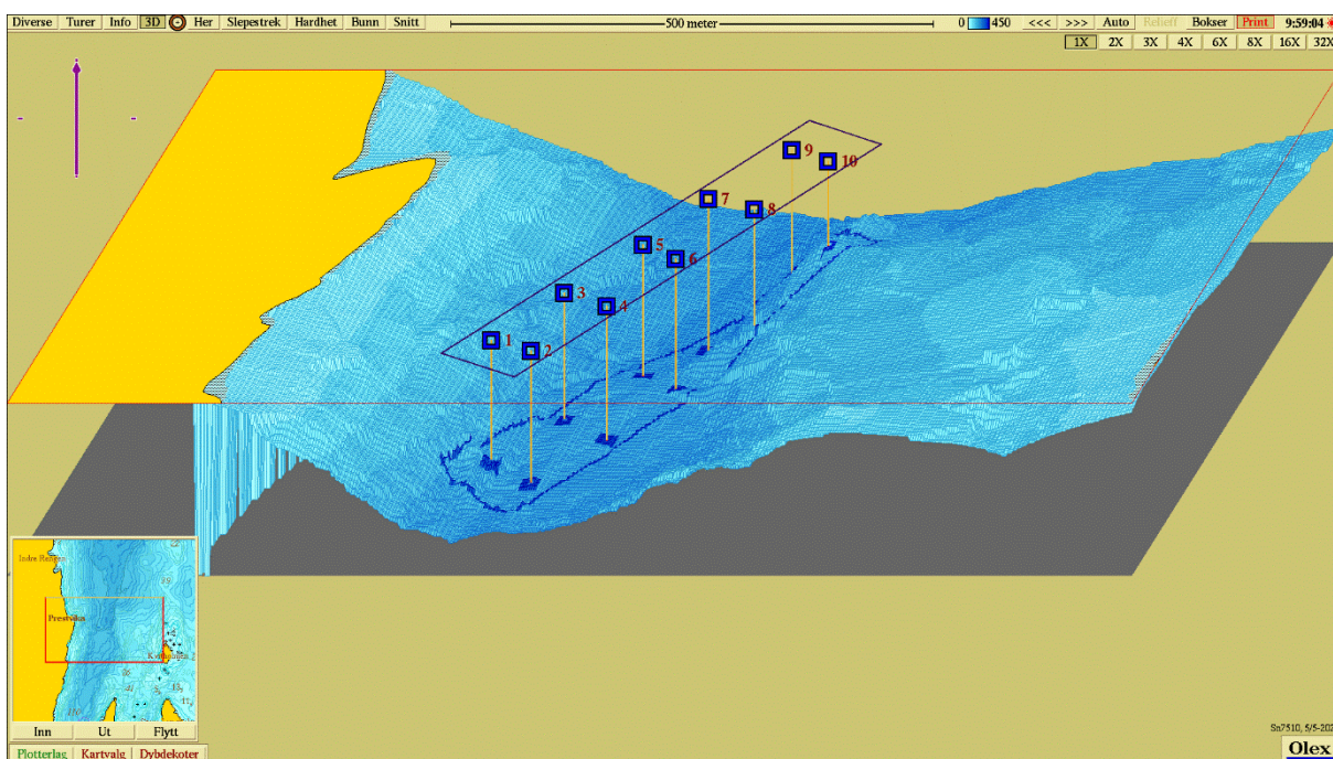
Figur 4: Tredimensjonalt isometrisk bunnskart med anleggsomriss og stasjoner. Stasjonene er markert med farge etter hva slags tilstand de har jmfør Tabell 8 . Målestokk vises øverst i bildet. Kartdatum WGS84. Kilde: Olex.
