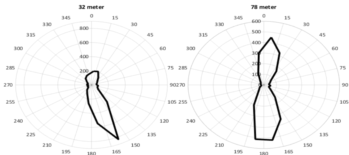
Figur 4: Vanntransport ( \text{m}^3/\text{m}^2/\text{dag} ) for hver 15^\circ sektor på hhv. 32 og 78 meters dyp ved Prestvika i perioden 04.04.2023–10.05.2023 (Nergaard, 2023).
