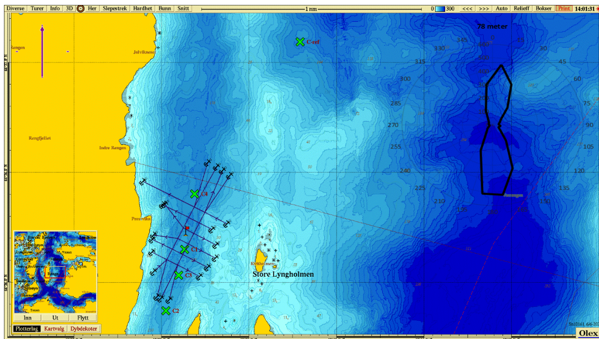
Figur 3.8: Anleggsplassering og strømforhold (vanntransport i m 3 /m 2 /døgn). Kartet angir hvordan anlegget er plassert og prøvetakingsstasjoner (grønne kryss). Spredningsstrøm er målt ved 78 m, enkelt rødt flagg viser plassering av strømmåler for 5, 15, 32, 78 og 138 meters dyp.
