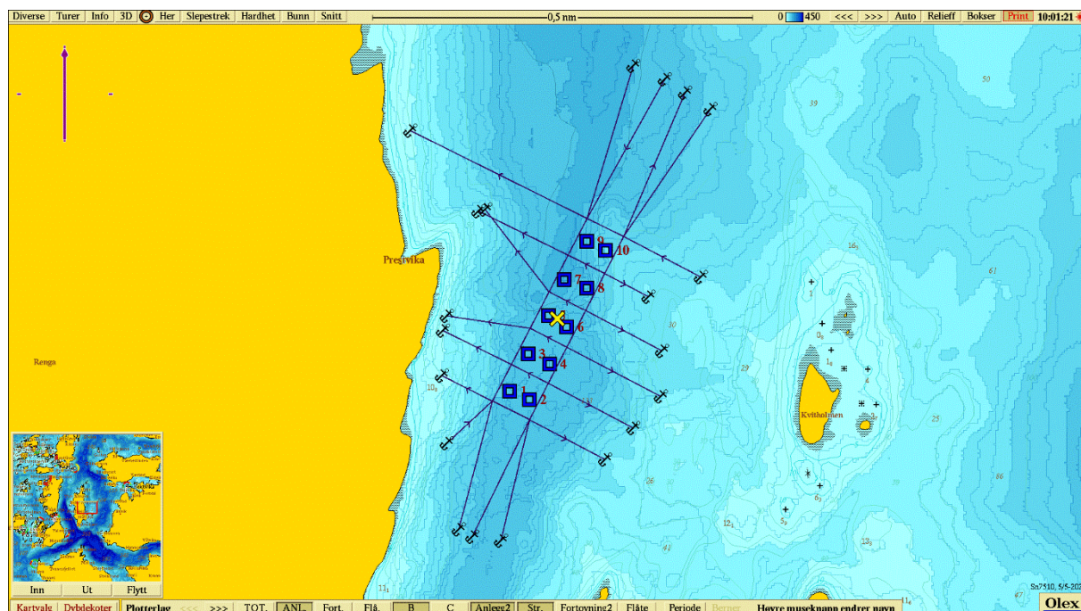
Figur 3.7: Kartet viser anleggs plassering sammen med B-stasjoner og fortøyningslinjer. Lilla pil viser orientering av kart, og gult kryss markerer posisjon for strømmålingene i 2021 ( 65^{\circ}15.450 N, 12^{\circ}14.150 Ø og 65^{\circ}15.477 N, 12^{\circ}14.023 Ø; Nergaard, 2023). Målestokk vises øverst i bildet. Kilde: Olex. Kartdatum WGS84.
