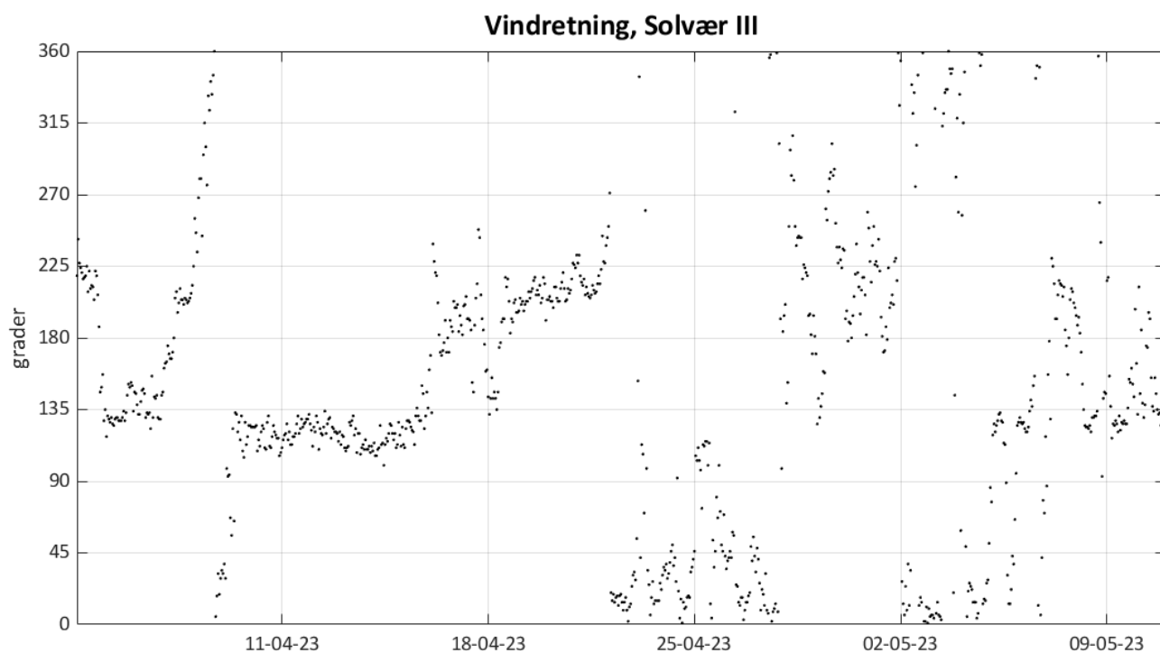
Figur B.2: Vindretning (°) ved den meteorologiske stasjonen Solvær III for perioden 04.04.–10.05.2023. Oppgis som retningen vinden blåser fra. Vindretningene er midlet over 1 time.
