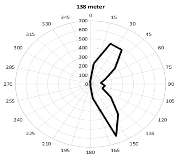
Figur 5: Vanntransport ( \text{m}^3/\text{m}^2/\text{dag} ) for hver 15^\circ sektor på 138 meters dyp ved Prestvika i perioden 04.04.2023–10.05.2023 (Nergaard, 2023).
