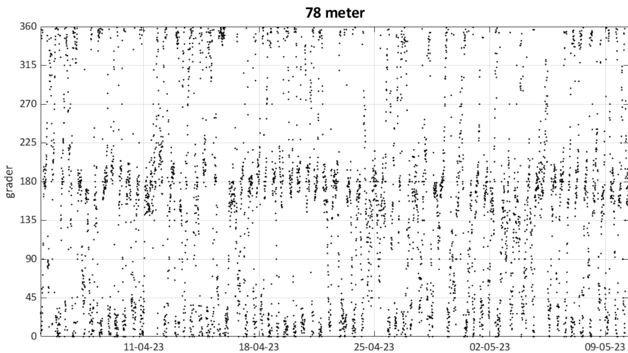
Figur 11: Vannstrømretning (°) på 78 meters dyp ved Prestvika i perioden 04.04.–10.05.2023. Oppgis som retningen vannstrømmen beveger seg mot.
