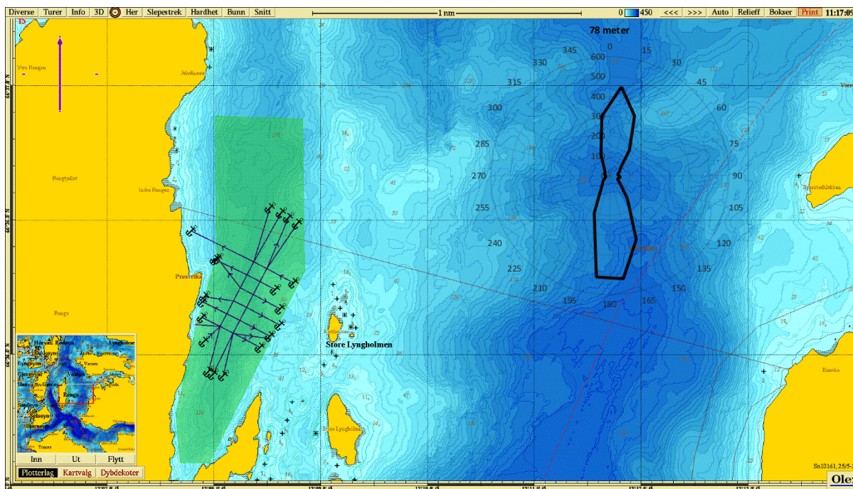
Figur 3.1: Planlagt anleggsplassering ved Prestvika. Det vurderte området er illustrert med grønt felt, strømrose viser vanntransport ( \text{m}^3/\text{m}^2/\text{dag} ) for hver 15° sektor på 78 meters dyp ved Prestvika i perioden 04.04.–10.15.2023 (Nergaard, 2023). Kilde: Olex. Kartdatum: WGS84.
