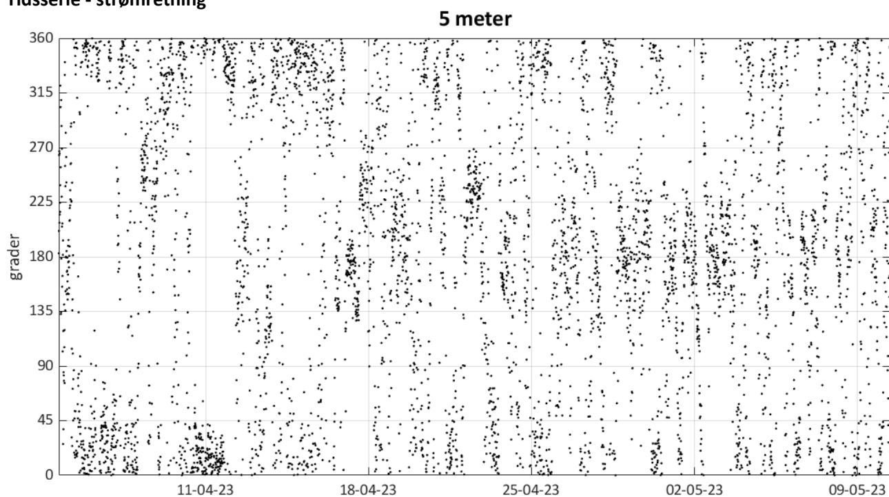
Figur B-6: Vannstrømretning (°) på 5 meters dyp ved Prestvika i perioden 04.04.–10.05.2023. Oppgis som retningen vannstrømmen beveger seg mot (Nergaard, 2023).
