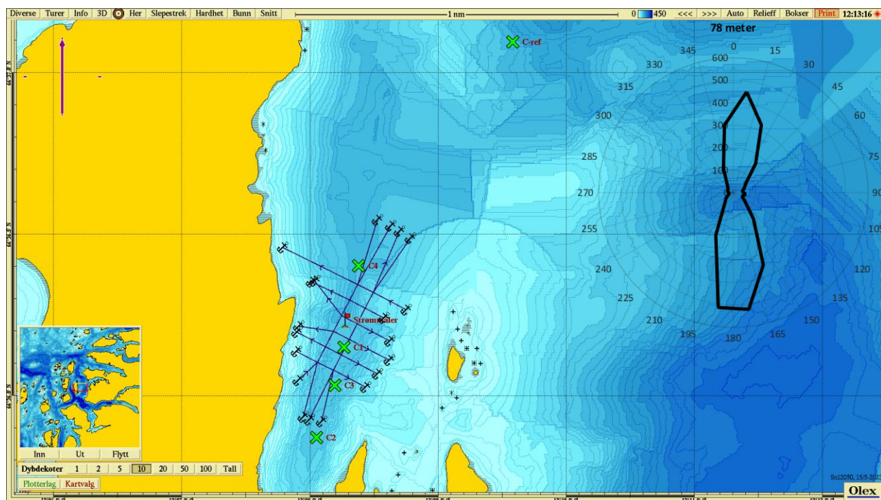
Figur 2: Anleggs plassering og strømforhold (vanntransport i m^3/m^2/døgn ). Kartet angir hvordan anlegget er plassert og prøvetakingsstasjoner. Spredningsstrøm er målt ved 78 m, og rødt flagg viser plassering av strømmåler. Kilde: Olex.
