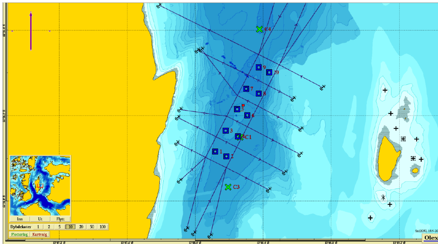
Figur 5: Sjøkart som viser bunndata fra Prestvika med planlagt anleggsplassering og fortøyningslinjer sammen med prøvestasjoner fra B-undersøkelsen (tilstand markert med farger etter Tabell 2) og C-undersøkelsens innerste stasjoner (grønne kryss). Lilla pil viser orientering av kart. Kilde: Olex. Kartdatum: WGS84.
