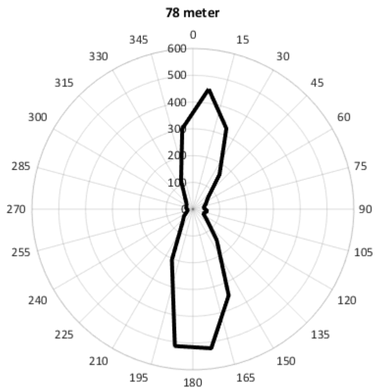
Figur 41: Vanntransport (m³/m²/dag) for hver 15° sektor på 78 meters dyp ved Prestvika i perioden 04.04.–10.05.2023.
