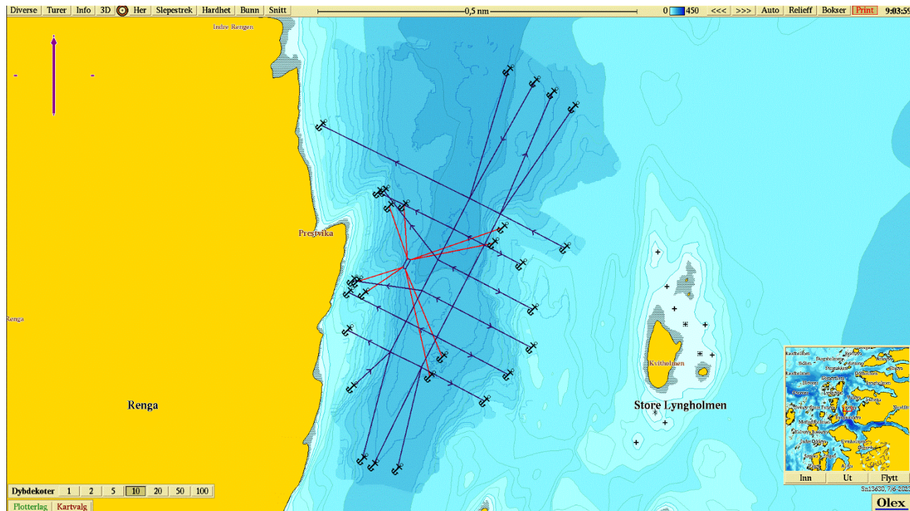
Figur 4.1.2: Oversiktskart over området med fortøyninger ved Prestvika. Dybdekoter for hver 10. meter er markert, og blåtoner fra lys til mørk markerer økende dybde. Målestokk vises øverst i figuren. Kartkilde: Olex.
