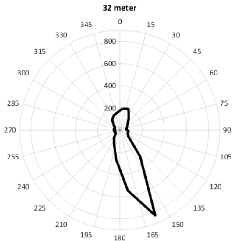
Figur 40: Vanntransport (m³/m²/dag) for hver 15° sektor på 32 meters dyp ved Prestvika i perioden 04.04.–10.05.2023.
