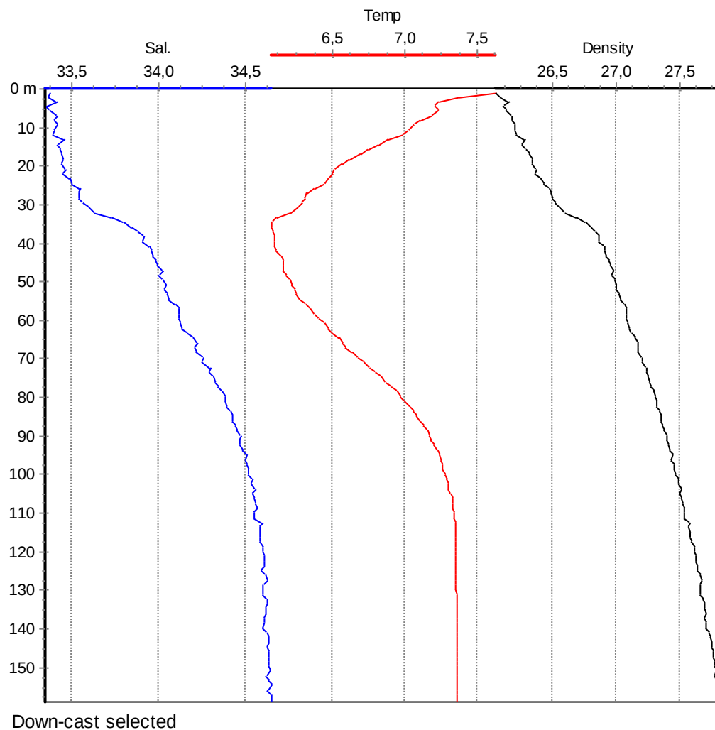
Figur 6: Sjøtemperatur (°C ; rød), salinitet (blå) og tetthet (-1000 kg/m³; sort) fra overflaten og ned til bunnen (down-cast) på 159 meters dyp ved stasjon C4 den 10.05.2023.
