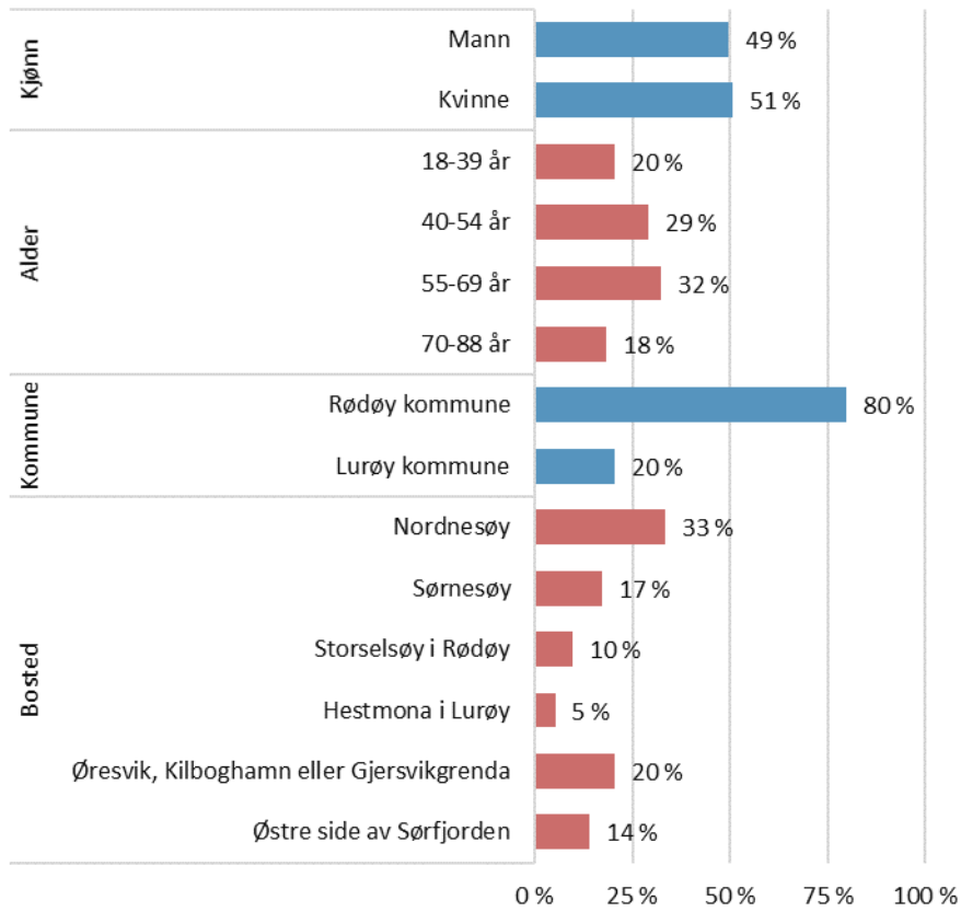
Figur 2: Bakgrunnsvariabler
