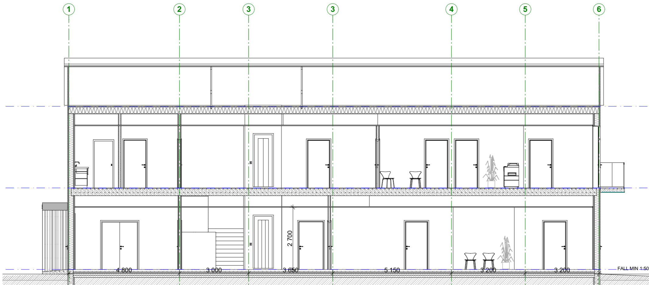
1:100 Snitt B
