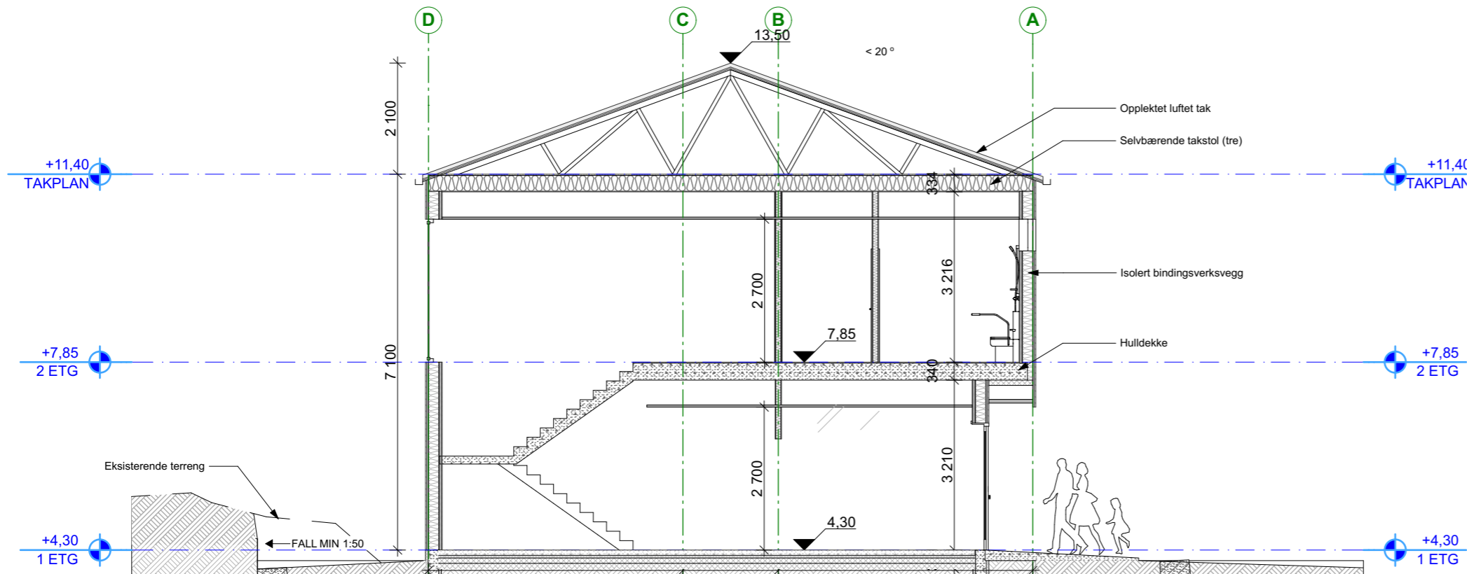
1:100 Snitt A
