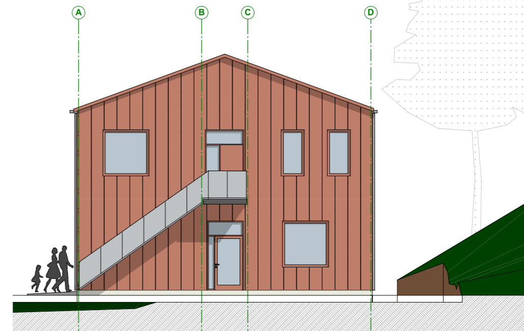
1:150 Fasade Nordøst
