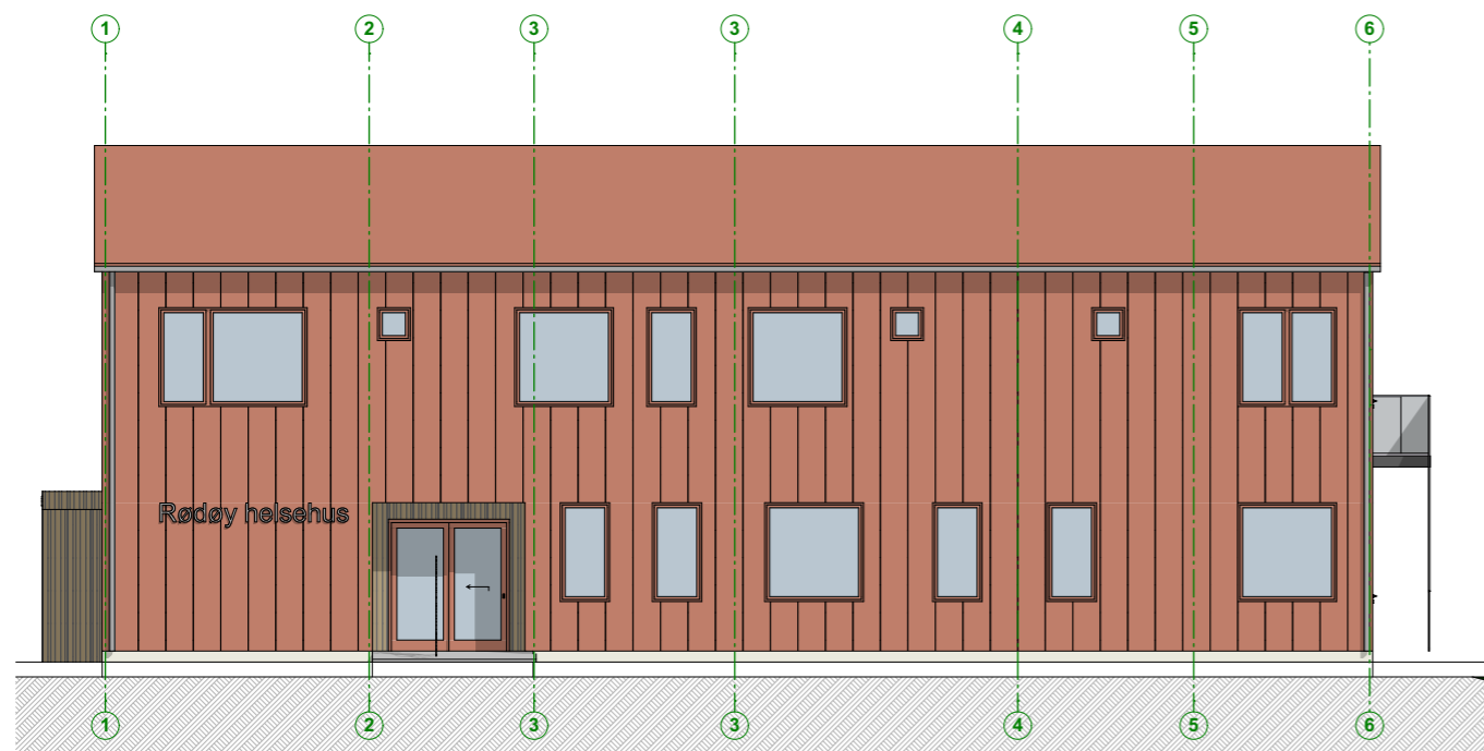
1:150 Fasade Sørøst
