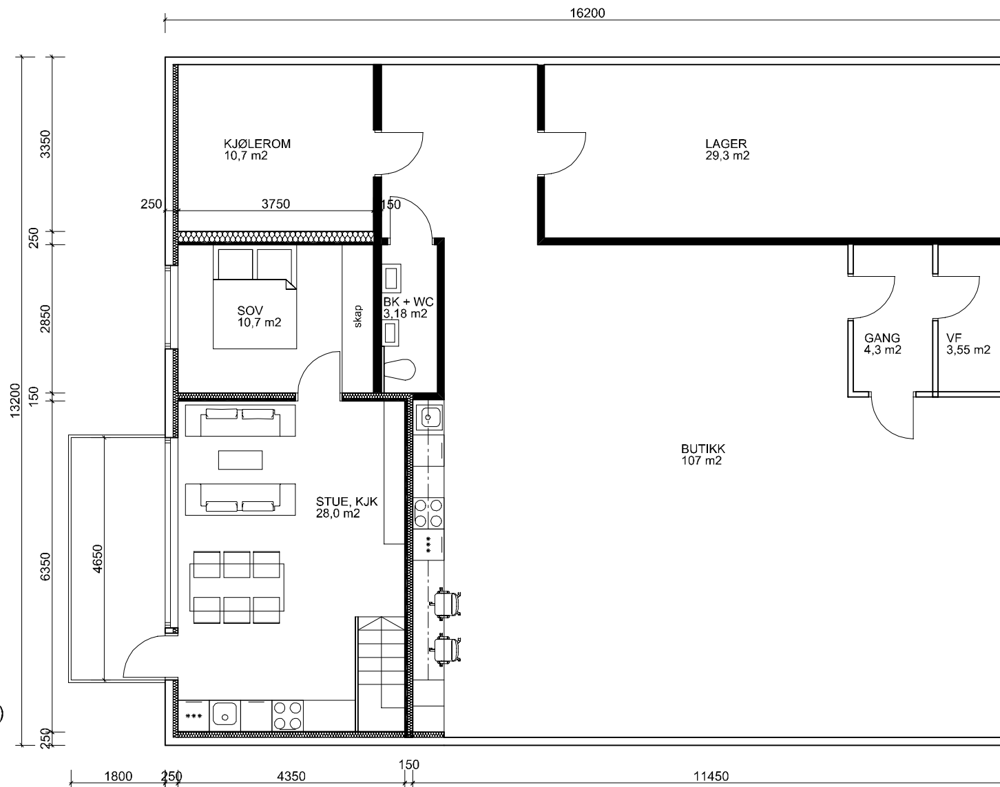
PLAN 1.ETASJE (Leil.) BRA 38,8 m 2
