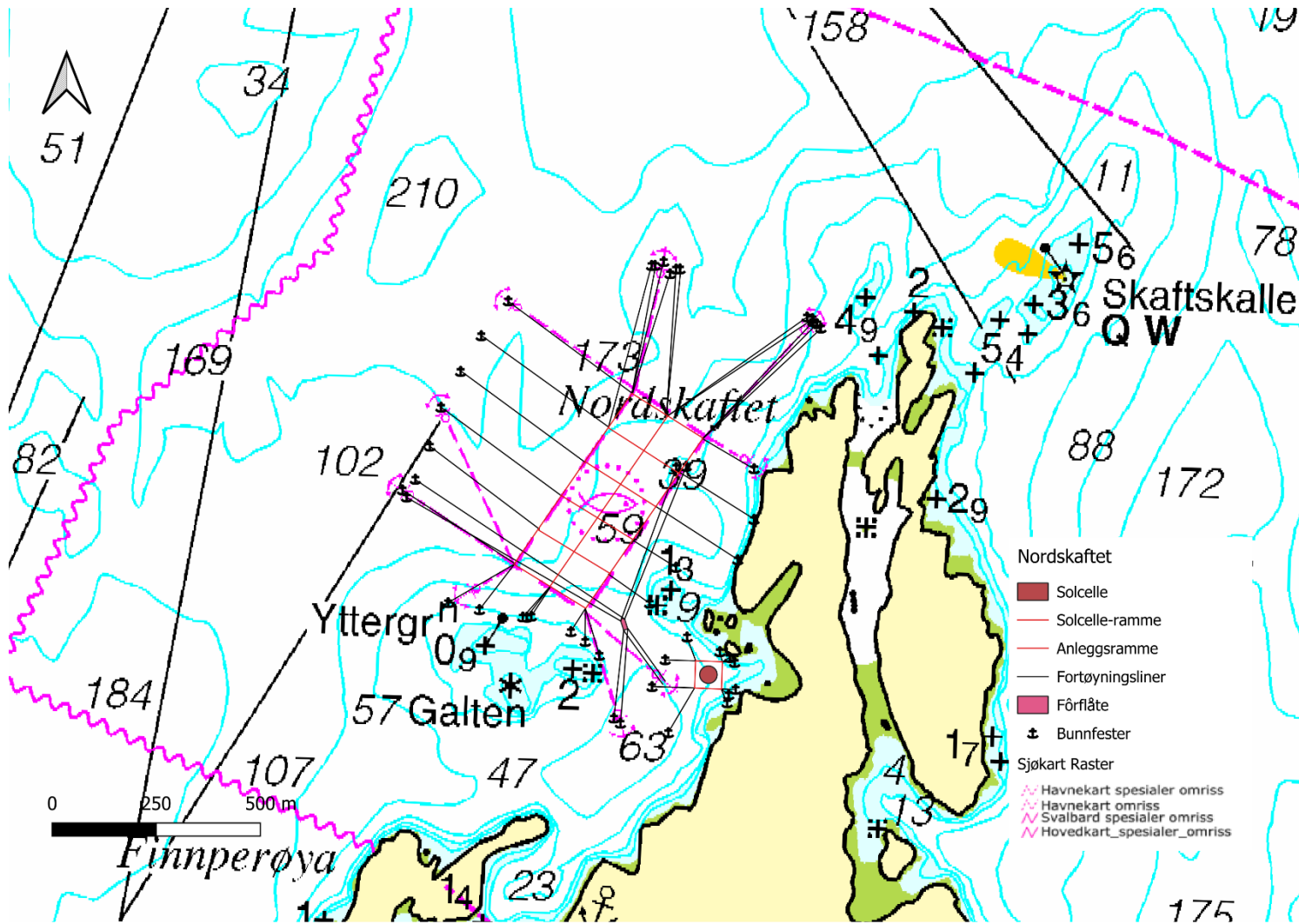
Figur 4: Sjøkart, anlegget ligger ikke i hvit sektor. Kilde: Kystverkets WMS.
