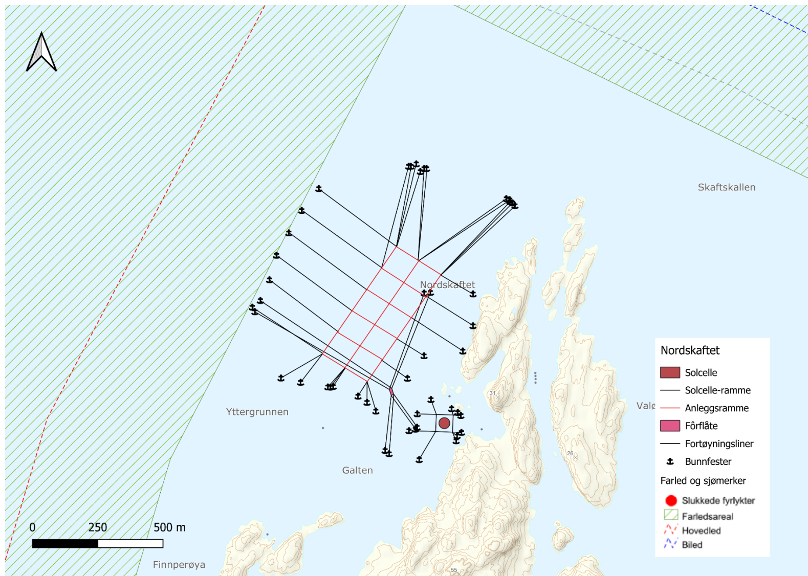
Figur 5: Farled, anlegget er ikke i konflikt med farledsareal, hovedled eller biled. Kilde: Kystverkets WMS.
