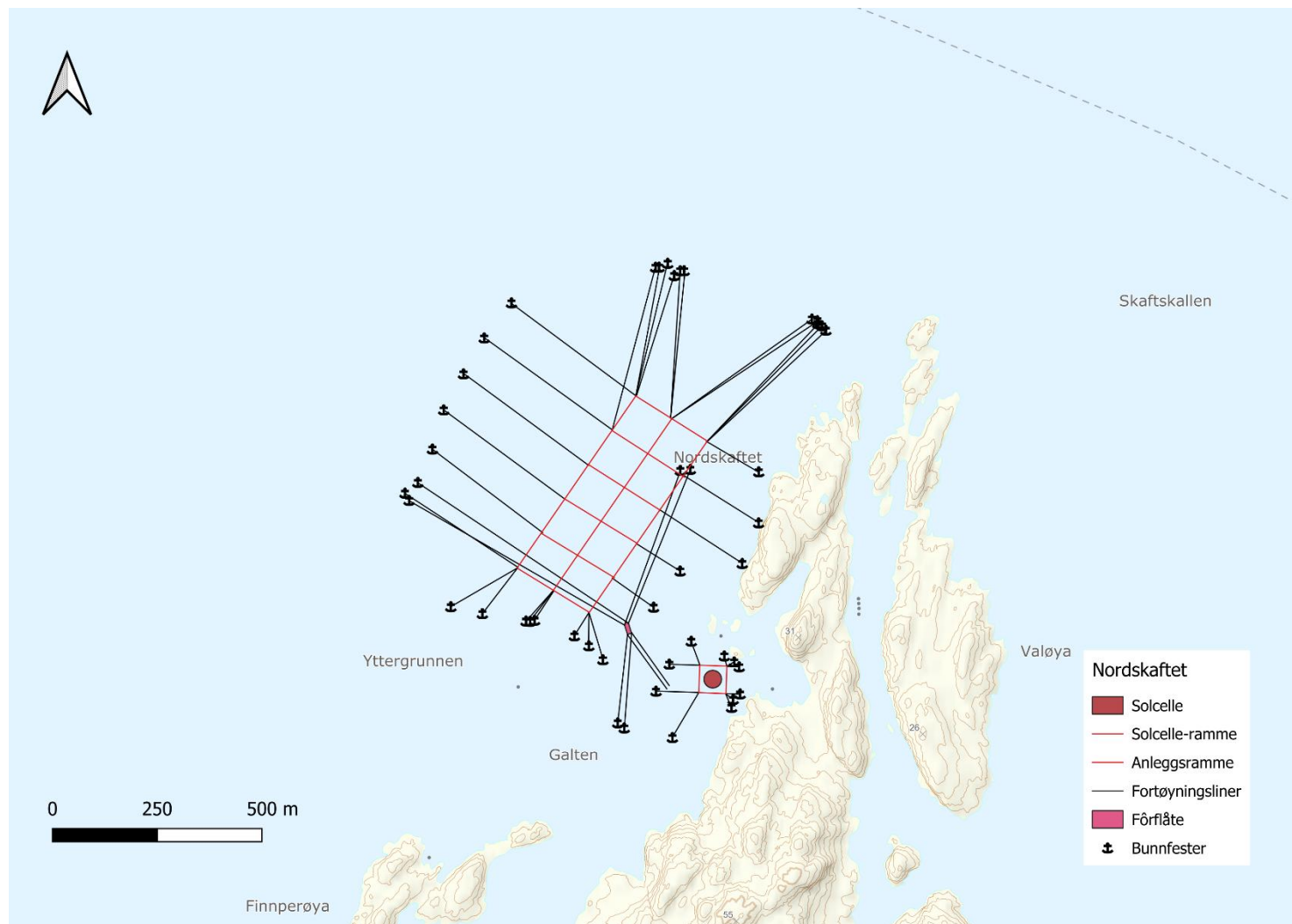
Figur 1: Illustrasjon av anlegget slik det ligger i dag og plassering av solcelle med fortøyninger.
